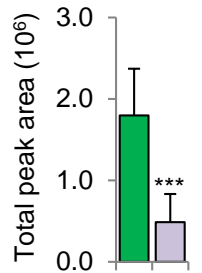
VTNC_HUMAN DVWGIEGPIDAAFR
