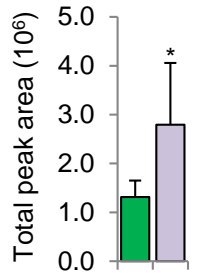
CO1A2_HUMAN GEIGAVGNAGPAGPAGPR
