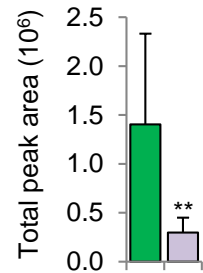
PGCA_HUMAN EVLLVATEGR
