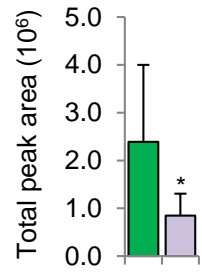
ASPN_HUMAN SLYSAISLFNNPVK
