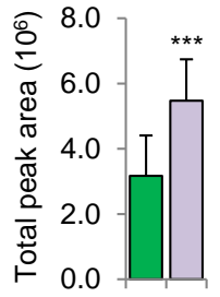
LAMC1_HUMAN LSAEDLVLEGAGLR
